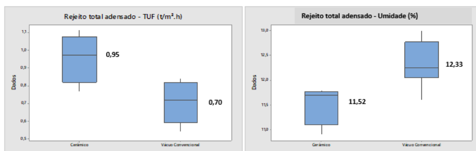
Figura 5. Resultados de TUF (t/m 2 .h) e umidade (%) para os testes de filtragem com rejeito total adensado.
