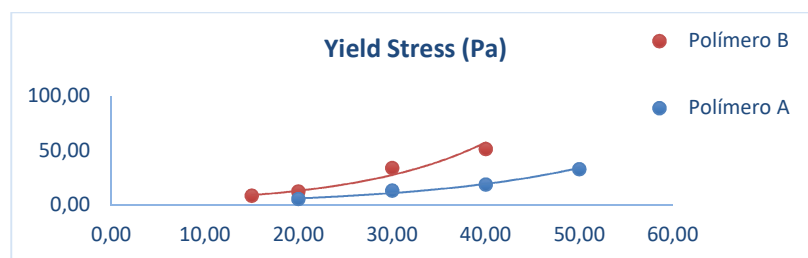
Figura 1. Comparativo Yield Stress (Pa).
