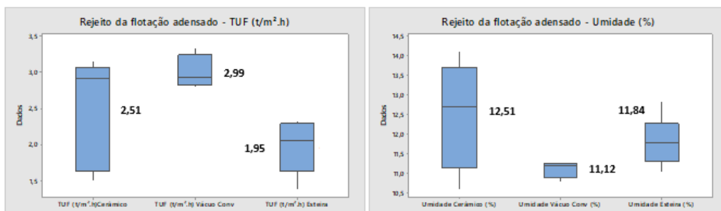
Figura 4. Resultados de TUF (t/m 2 .h) e umidade (%) para os testes de filtragem com rejeito da flotação adensado.
