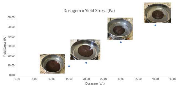
Figura 2. Testes para determinação da dosagem ideal.
